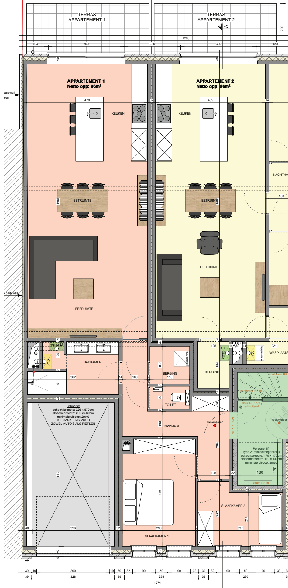
GELIJKVLOERS Schaal 1/50
